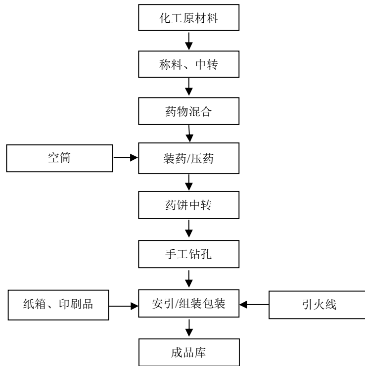
图 2-4：旋转类（大地花开）生产工艺流程图
