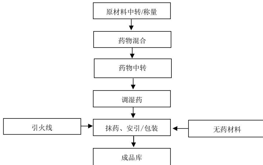
图 2-6：喷花类（闪光）产品生产工艺流程图
