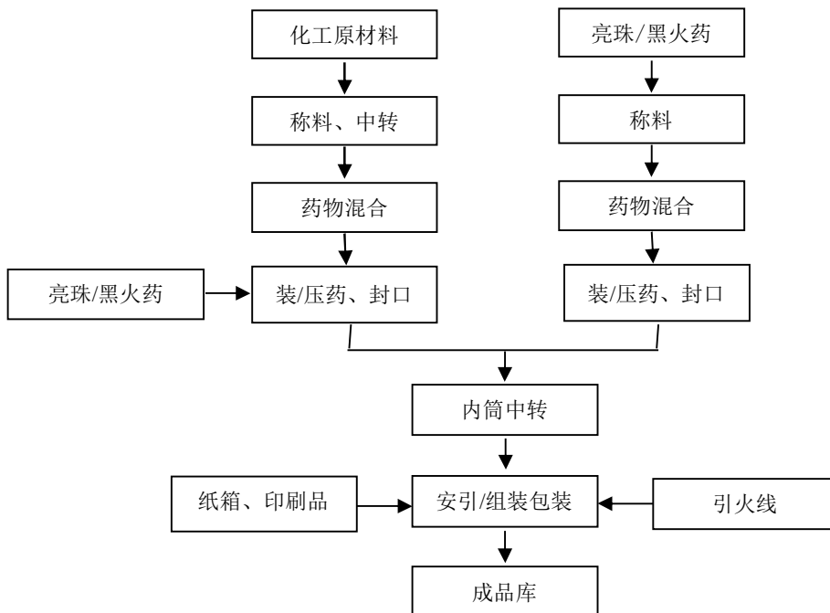
图 2-5：喷花类/玩具类（玩具造型）生产工艺流程图
