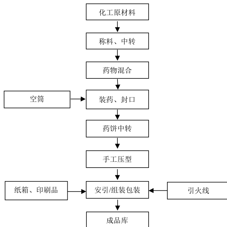
图 2-3：旋转类（茶花香）生产工艺流程图
