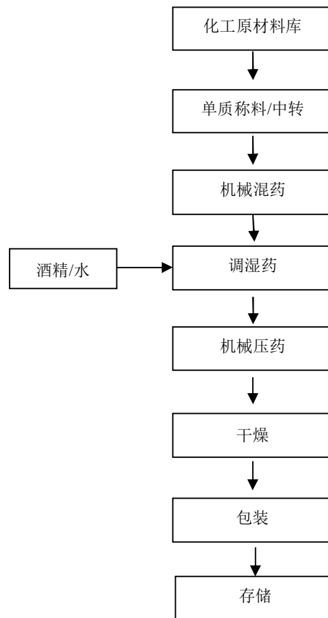
图 2-9：药柱生产工艺流程图
