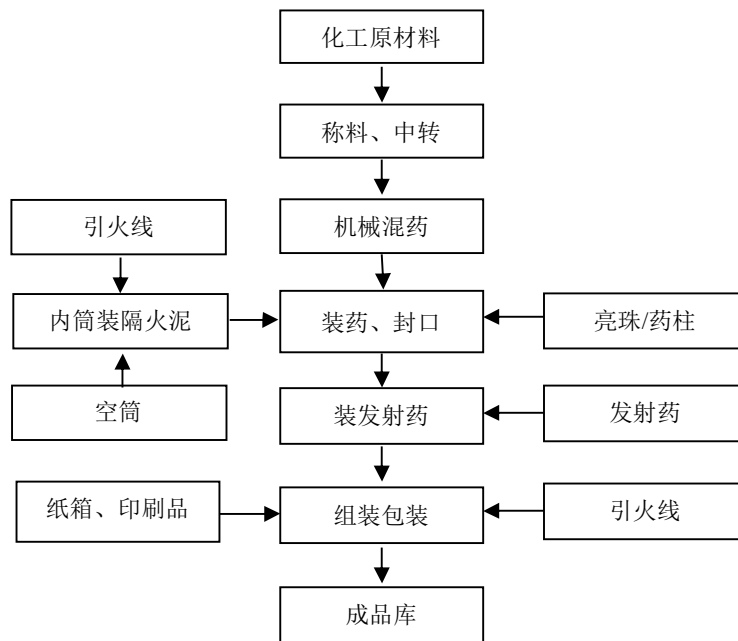
图 2-2：小礼花生产工艺流程图
