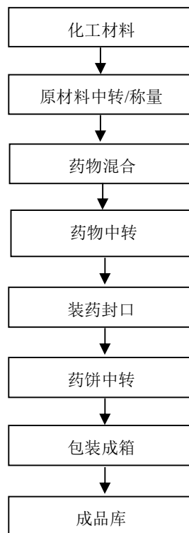
图 2-7：玩具类（线香型）产品生产工艺流程图
