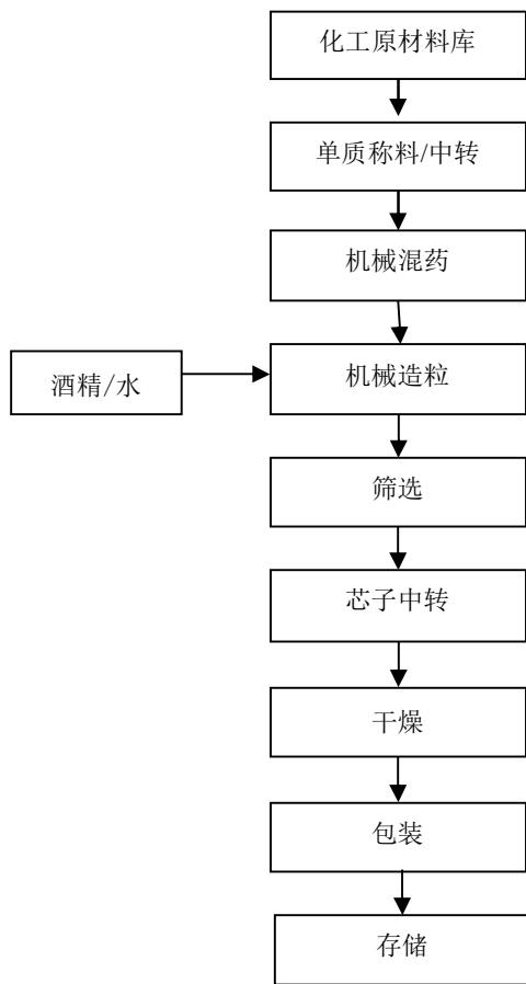
图 2-8：亮珠生产工艺流程图
