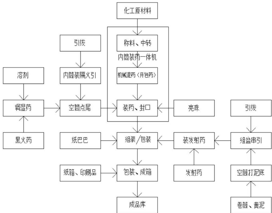
图 2-1：组合烟花类生产工艺流程图
