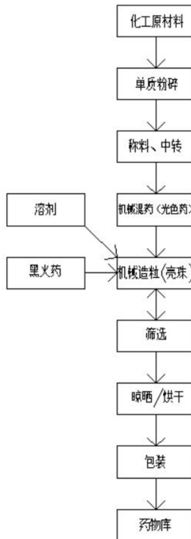
图 2-3：烟火药（亮珠）生产工艺流程图
