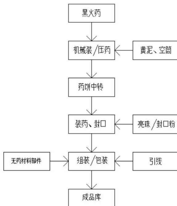
图 2-2：升空类（火箭）生产工艺流程图
